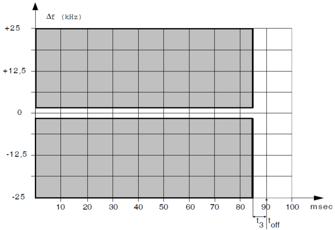
圖 1、DSC MSLD AU 發射機瞬時頻率行為之時序限制圖（參考 RTCM
