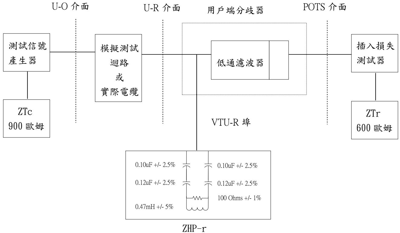
圖三 語音頻帶插入損失測試接線圖
