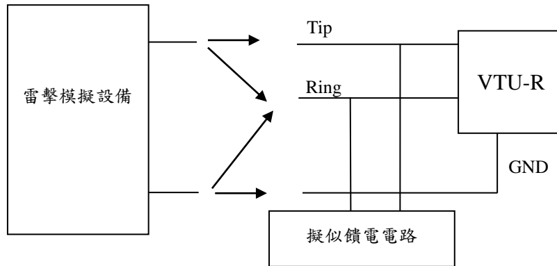
圖十六 U-R 介面雷擊試驗接線圖
