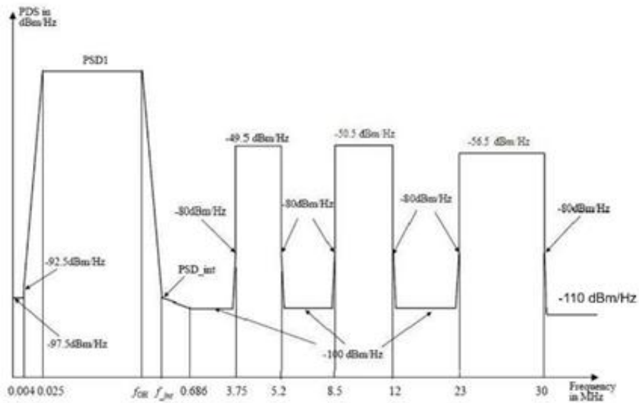
(3) Profile 30a的功率頻譜密度遮罩
