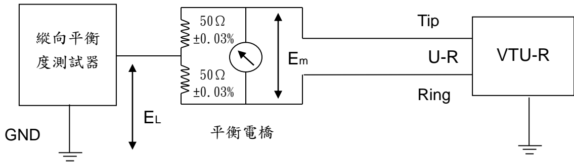
圖十四 縱向平衡度測試架構圖
