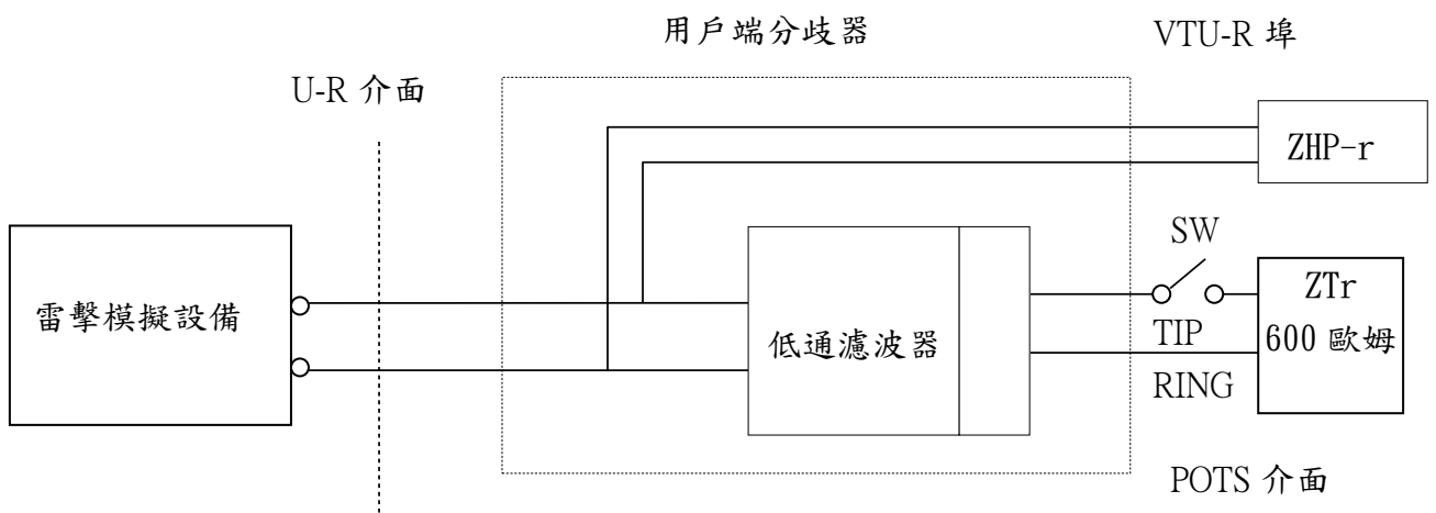
圖十一 雷擊試驗接線圖
