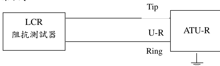
圖十五 ATU-R 輸入阻抗測試架構圖
