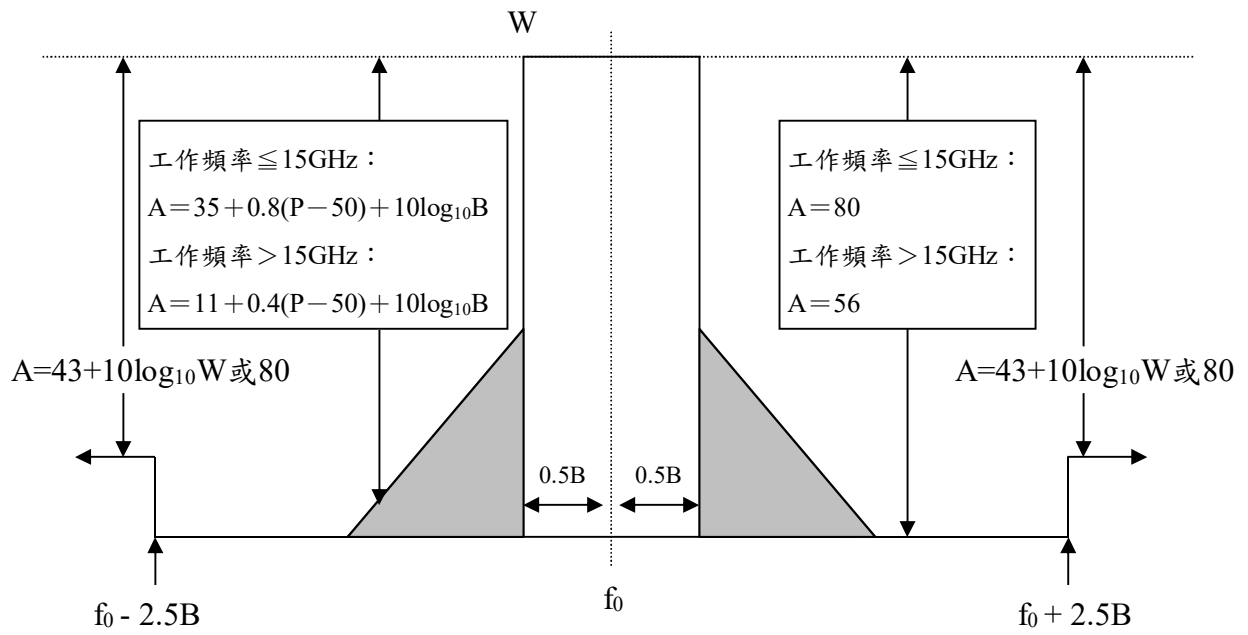
發射頻譜
