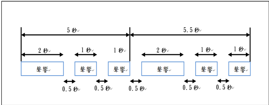
圖 4、告警聲響信號之圖示
