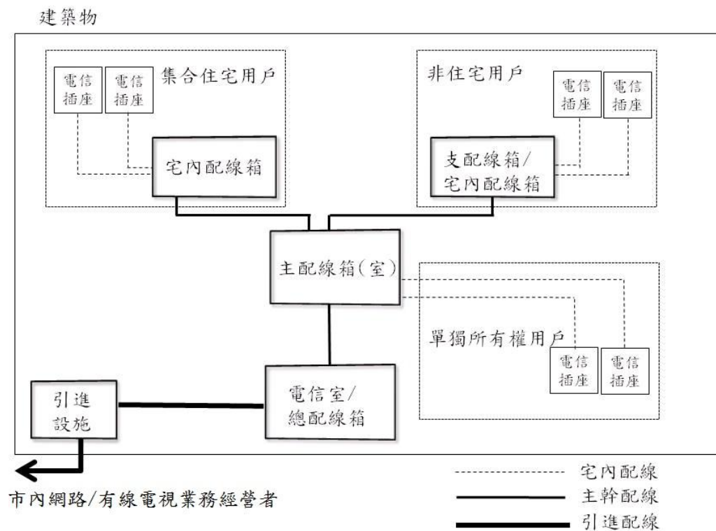
圖4-2 一般建築物電信設備架構圖
