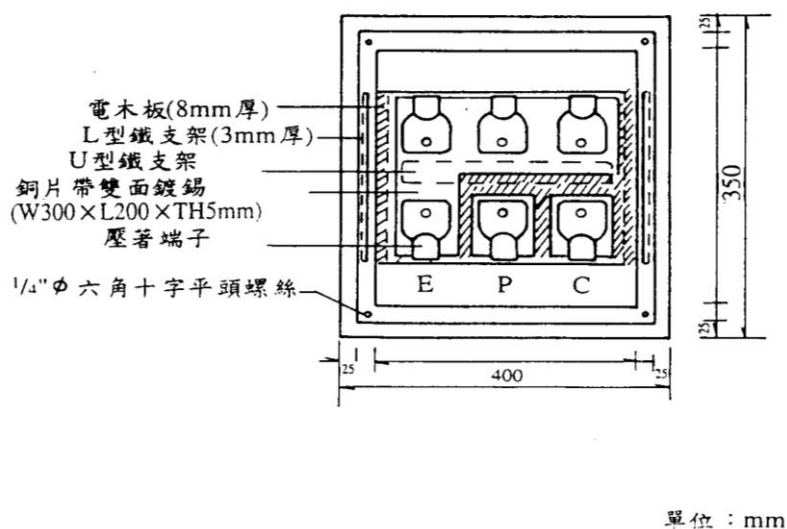
圖 14-1 總接地箱正視圖
