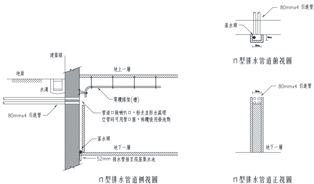
圖15-1 ㄇ型排水管道配置圖
