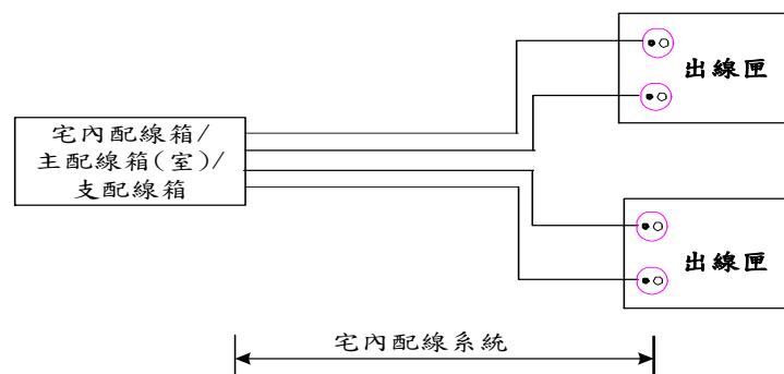
圖4-9 一般宅內配線系統架構圖
