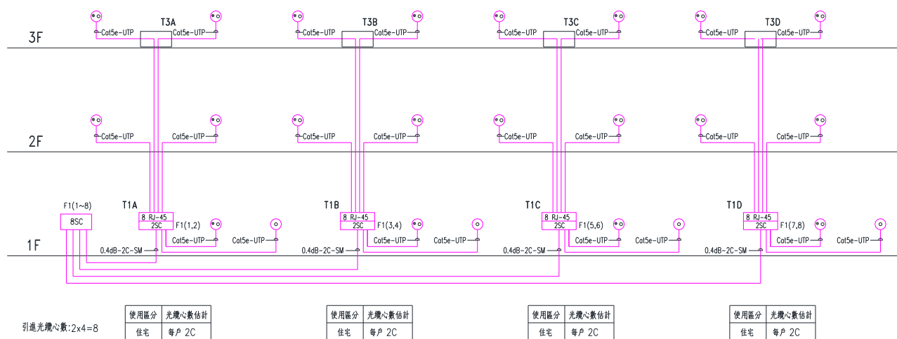
圖17-6 設計範例(二)光纜及資訊纜線昇位圖
