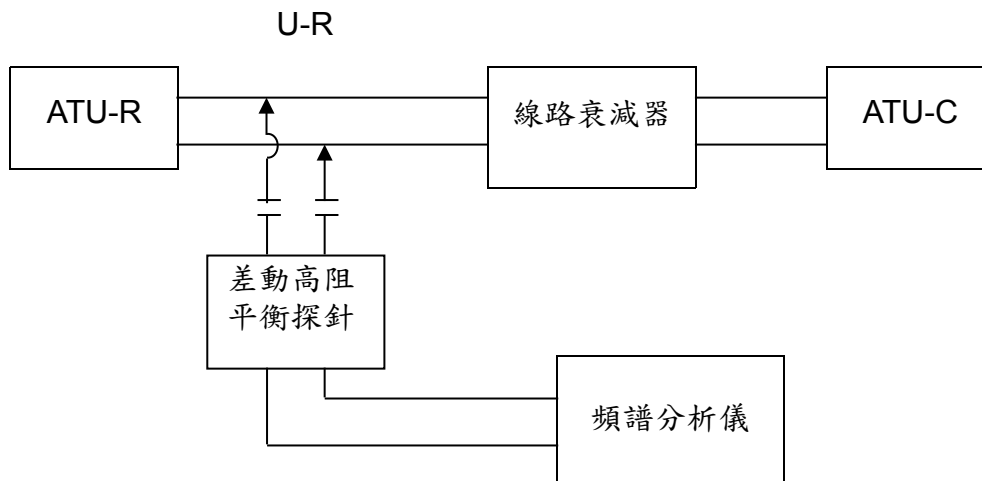
圖十二 ATU-R 發送信號功率頻譜密度測試架構圖
