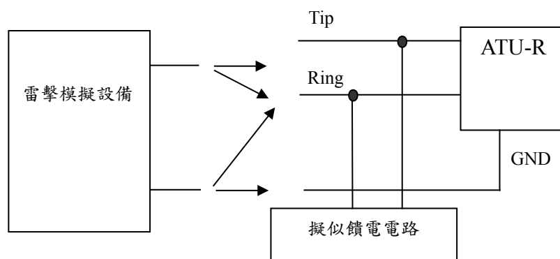
圖十六 電話線雷擊測試架構圖
