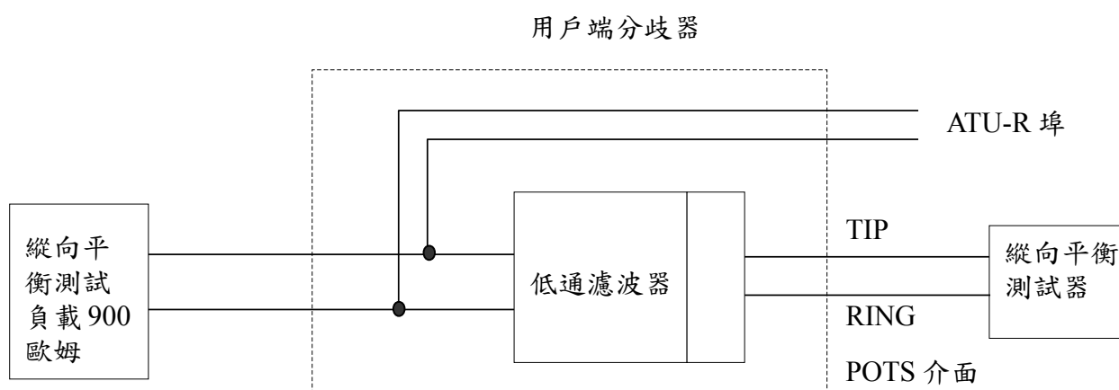
圖九 縱向平衡測試接線圖
