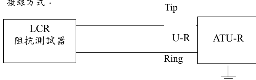
圖十五 ATU-R 輸入阻抗測試架構圖
