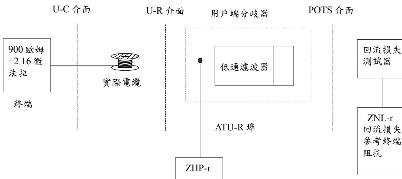
圖八 回流損失測試接線圖
