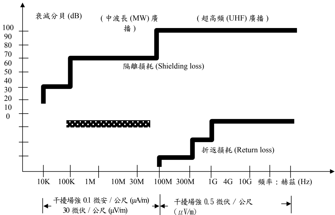
圖二：隔離室的幾何配置以及其隔離損耗與壁面折返損耗的規格需求
